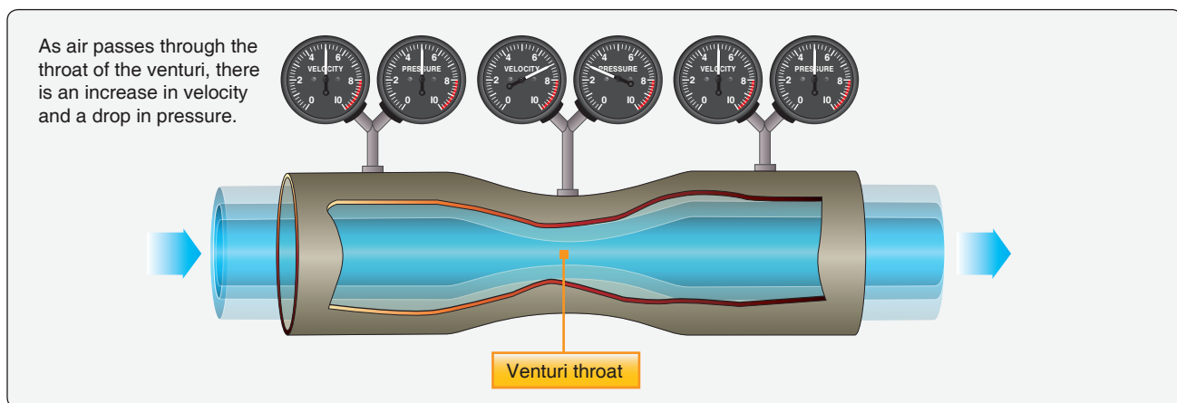
Figure 2-4. Simple venturi.
